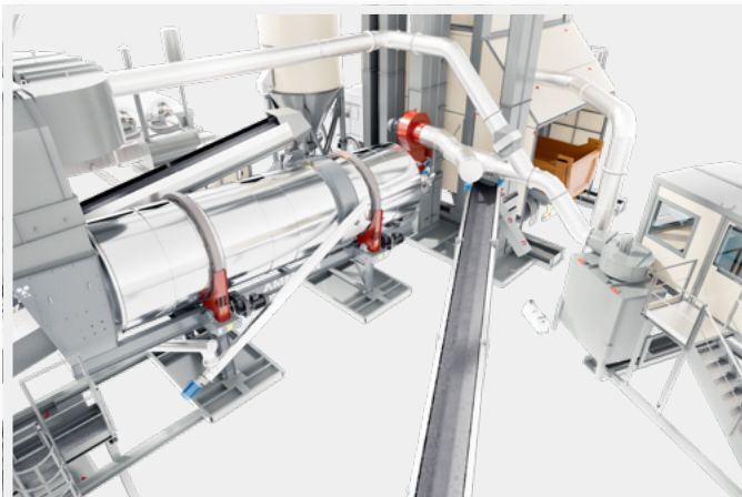
Les fumées bleues sont filtrées et nettoyées et l'air résultant est réutilisé dans le processus de séchage-chauffage
