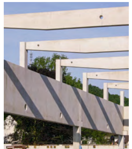
Poteaux et poutres
